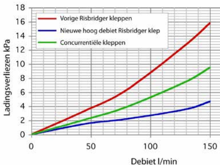
Ladingsverliezen (kPa) in functie van het Debiet (l/min)
